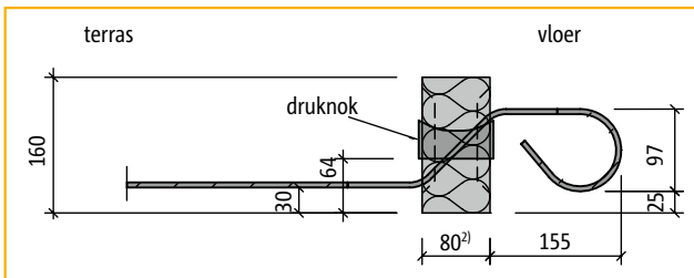
Schöck Isokorb® type Q10, Q30 en Q50 1)
