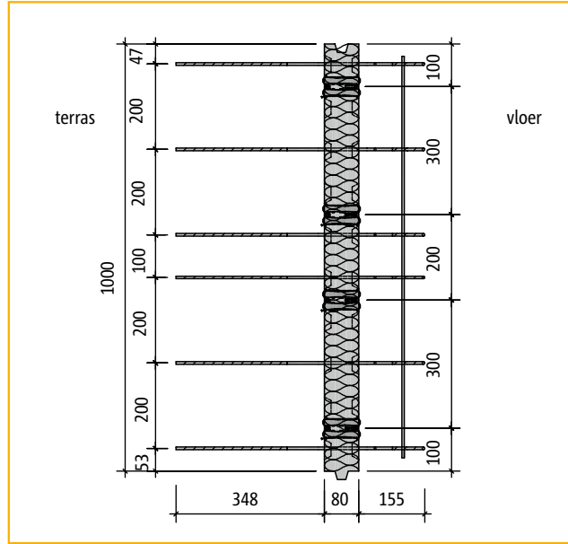
Bovenaanzicht Schöck Isokorb® type Q30 1)
