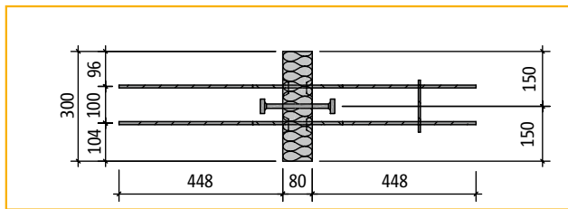
Bovenaanzicht Schöck Isokorb® type QP10 1)
