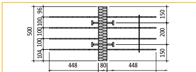
Bovenaanzicht Schöck Isokorb® type QP30 1)
