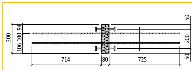
Bovenaanzicht Schöck Isokorb® type QP60 3)
