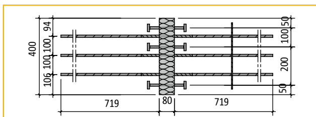
Bovenaanzicht Schöck Isokorb® type QP70 3)
