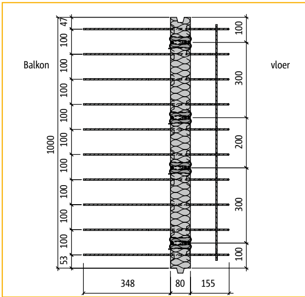
Bovenaanzicht Schöck Isokorb® type Q50 1)
