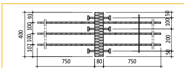
Bovenaanzicht Schöck Isokorb® type QP90 3)
