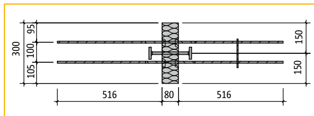
Bovenaanzicht Schöck Isokorb® type QP40 2)
