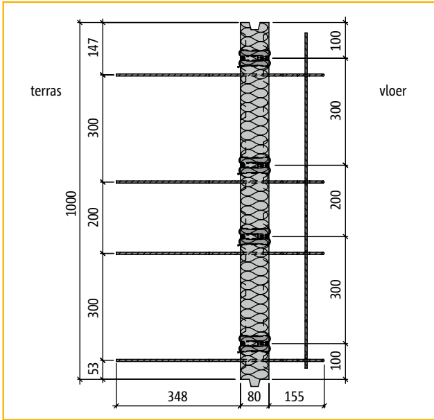
Bovenaanzicht Schöck Isokorb® type Q10 1)
