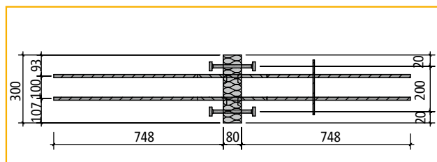
Bovenaanzicht Schöck Isokorb® type QP80 3)
