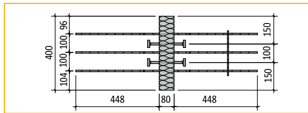
Bovenaanzicht Schöck Isokorb® type QP20 1)
