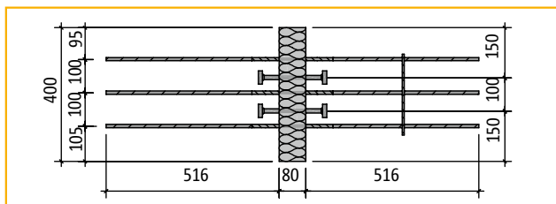
Bovenaanzicht Schöck Isokorb® type QP50 2)
