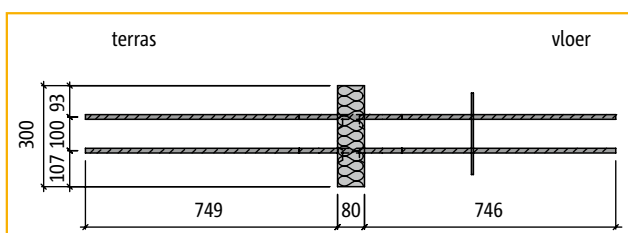
Bovenaanzicht Schöck Isokorb® type QPZ80 (Z=spanningsvrij)
